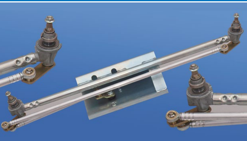
▶ Kundenspezifische Gleichläufer-Wischanlage mit Gelenkköpfen und Aluminium-Schubstangen
